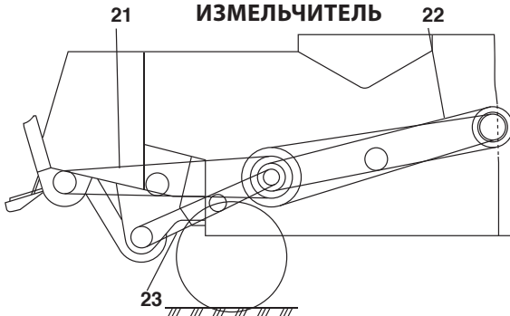
ИЗМЕЛЬЧИТЕЛЬ
